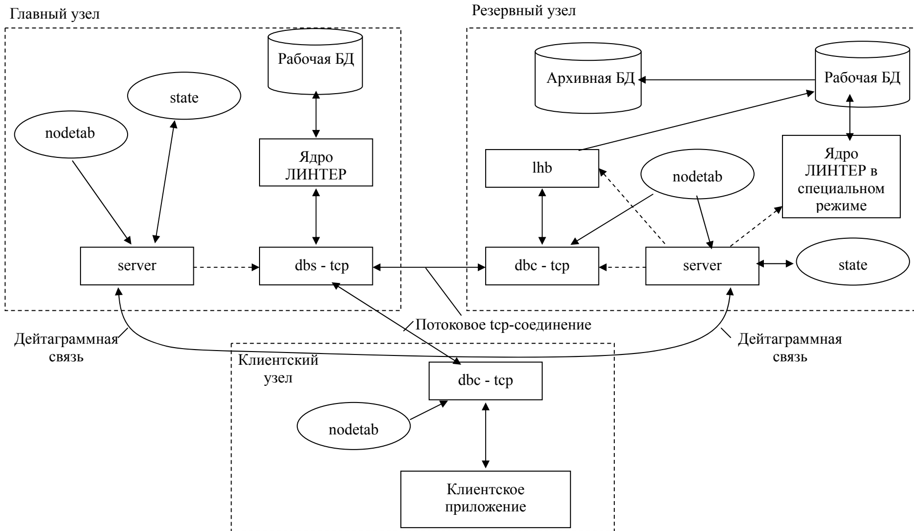
Рис. 2. Схема взаимодействия СУБД ЛИНТЕР и системы резервирования
